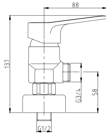
Toilet Mixer
