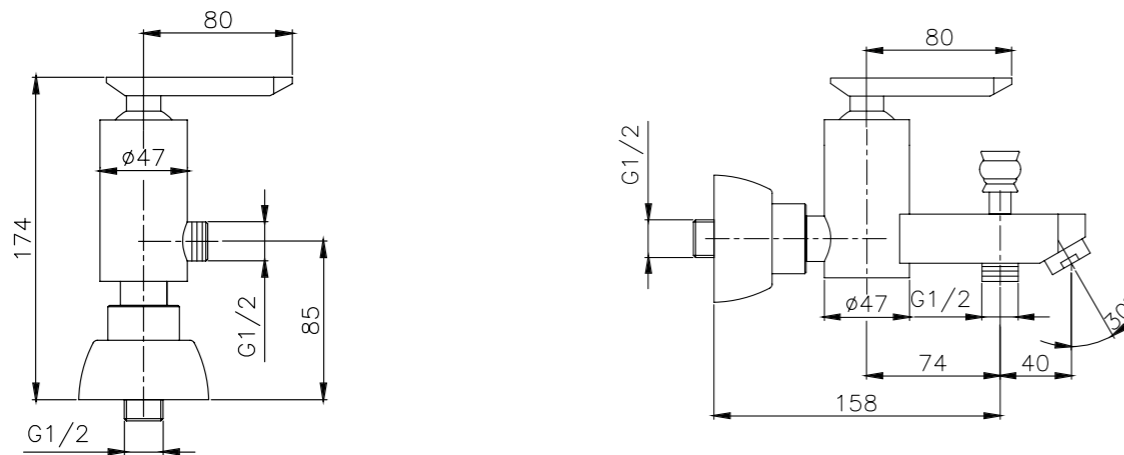
Toilet Mixer
