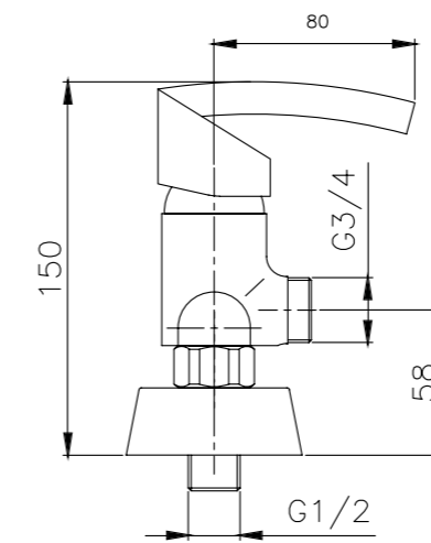
Toilet Mixer
